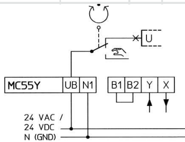
Schaltplan MC100 / MC160 / MC161
