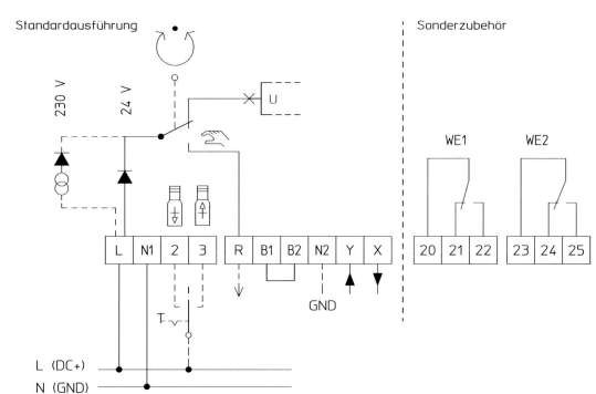
B1/B2 Anschlußmöglichkeit eines Binärsignals (z.B. Frostschutz)
