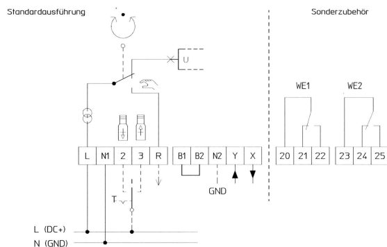
B1/B2 Anschlußmöglichkeit eines Binärsignals (z.B. Frostschutz)
