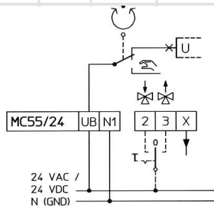
Schaltplan MC250 / MC500 / MC1000
