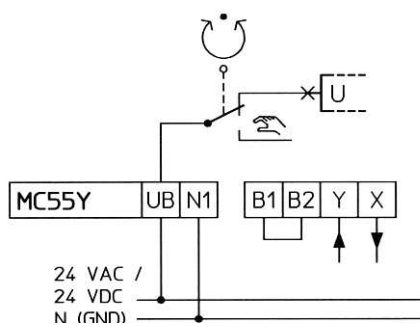
Schaltplan MC100 / MC160 / MC161
