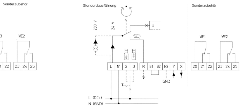
B1/B2 Anschlußmöglichkeit eines Binärsignals (z.B. Frostschutz)
